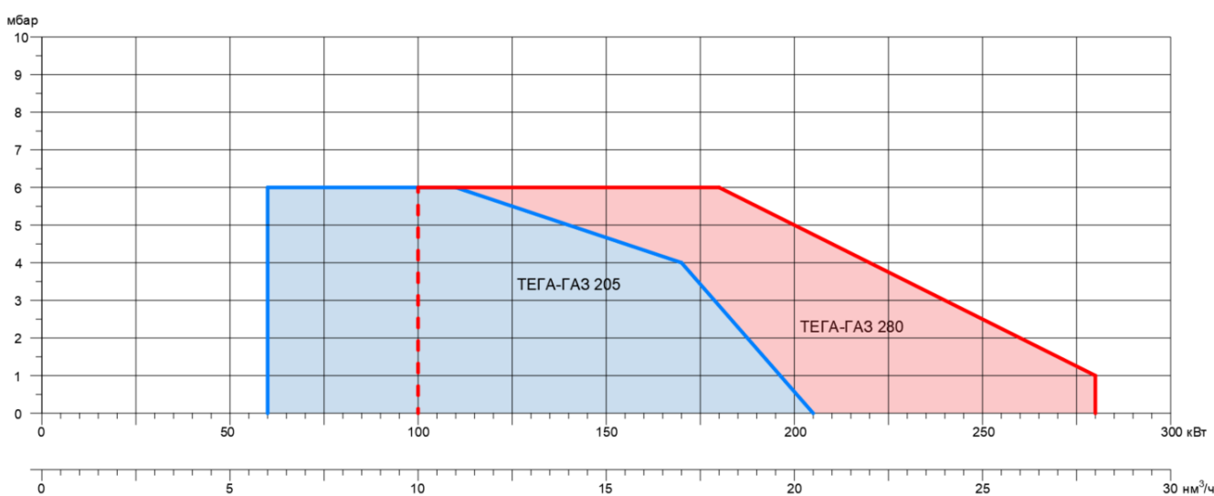
График рабочего поля горелок ТЕГА-ГАЗ 205.1 – 280.1
